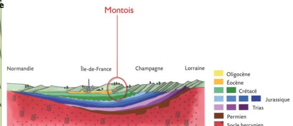
Coupe géologique simplifiée du bassin de Paris
